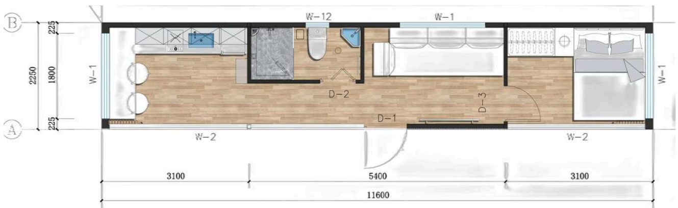
Orbit Suite, 2,25 × 11,60 m. Duo folgt demselben Querschnitt, anders geteilt.
